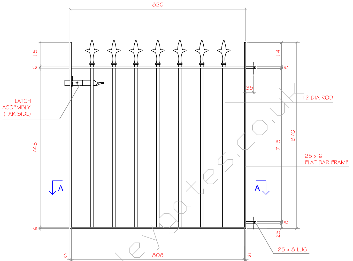
ELEVATION
